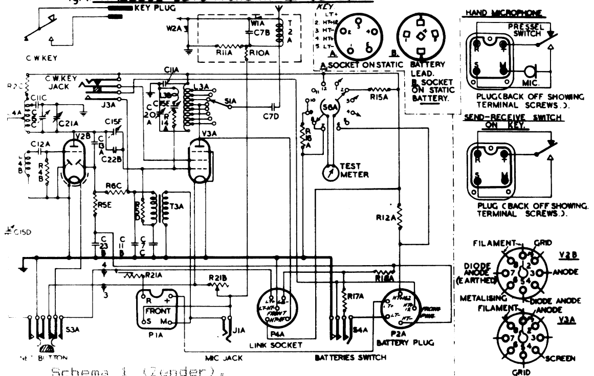
Schema 1 (Zender).
